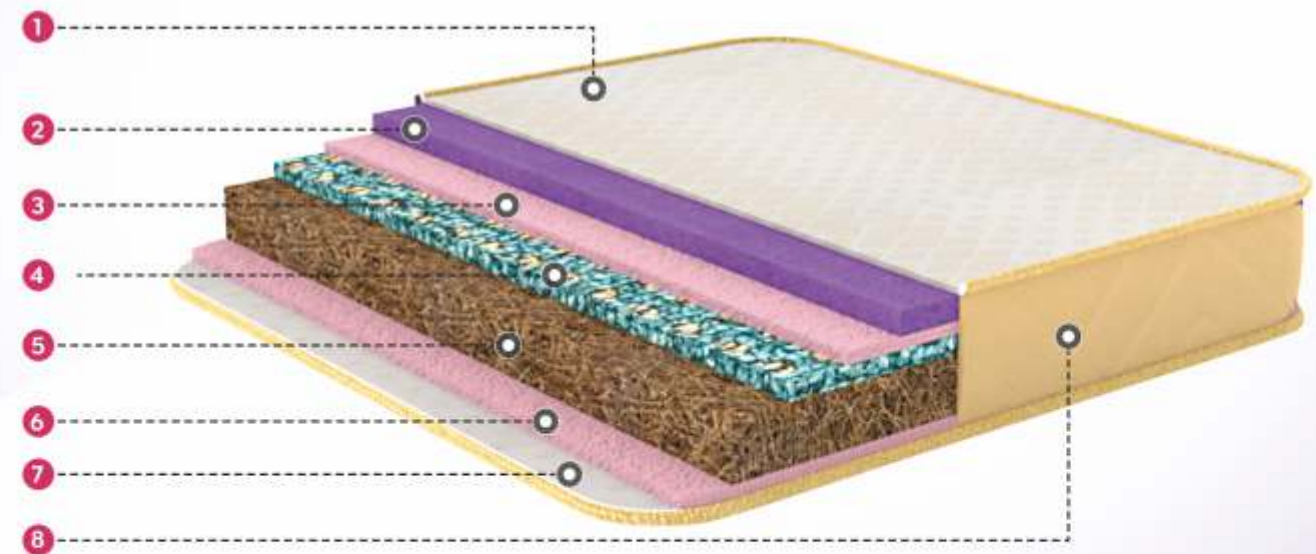
1. Fabric 2. Memory Foam 3. PU Foam 4. Bonded Foam 5. HD Coir 6. PU Foam 7. Fabric 8. Side Wall Quilt
